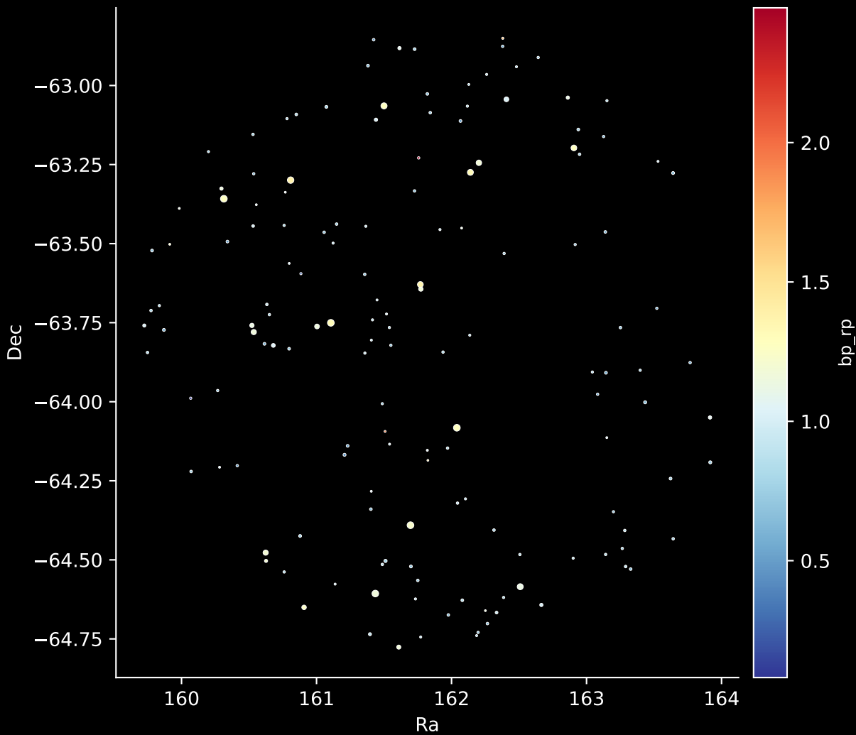
GALAH DR4 Field: [7210] Stars: 149
