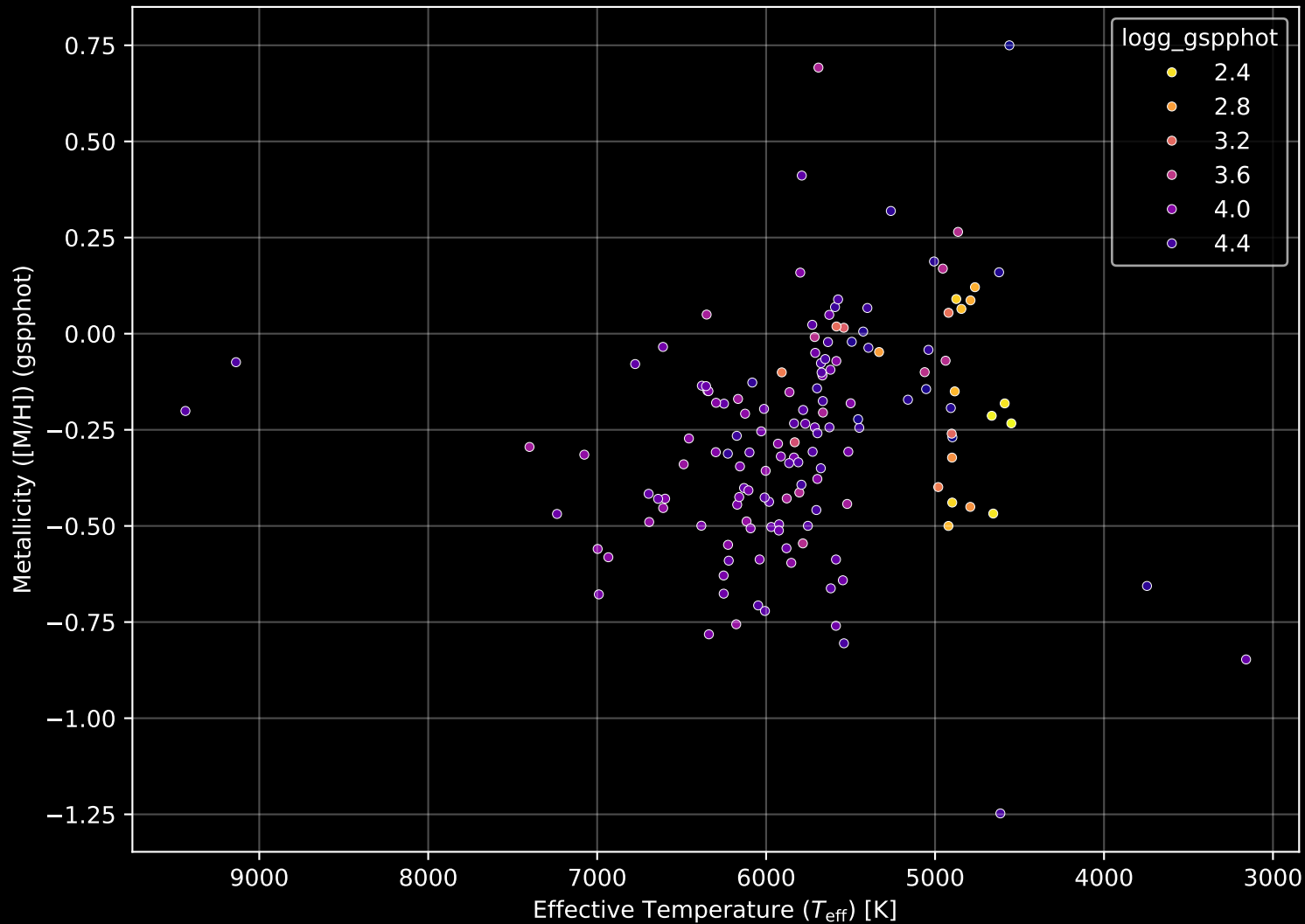
GALAH DR4 Field: [7210] Stellar Population Parameters (n= 149)
